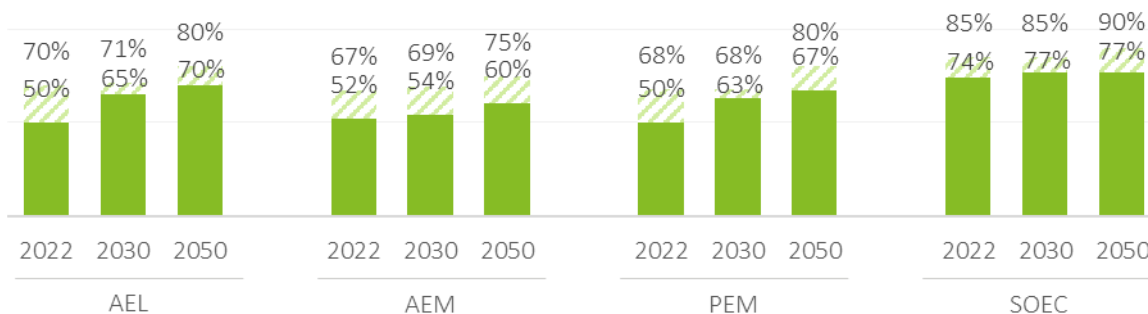
Ilustración 4 - Estimación de las eficiencias para varios tipos de electrolizadores 25
