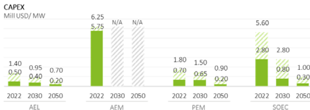
Ilustración 3 – Estimación de los costos de capital (CAPEX) para varios tipos de electrolizadores 25
